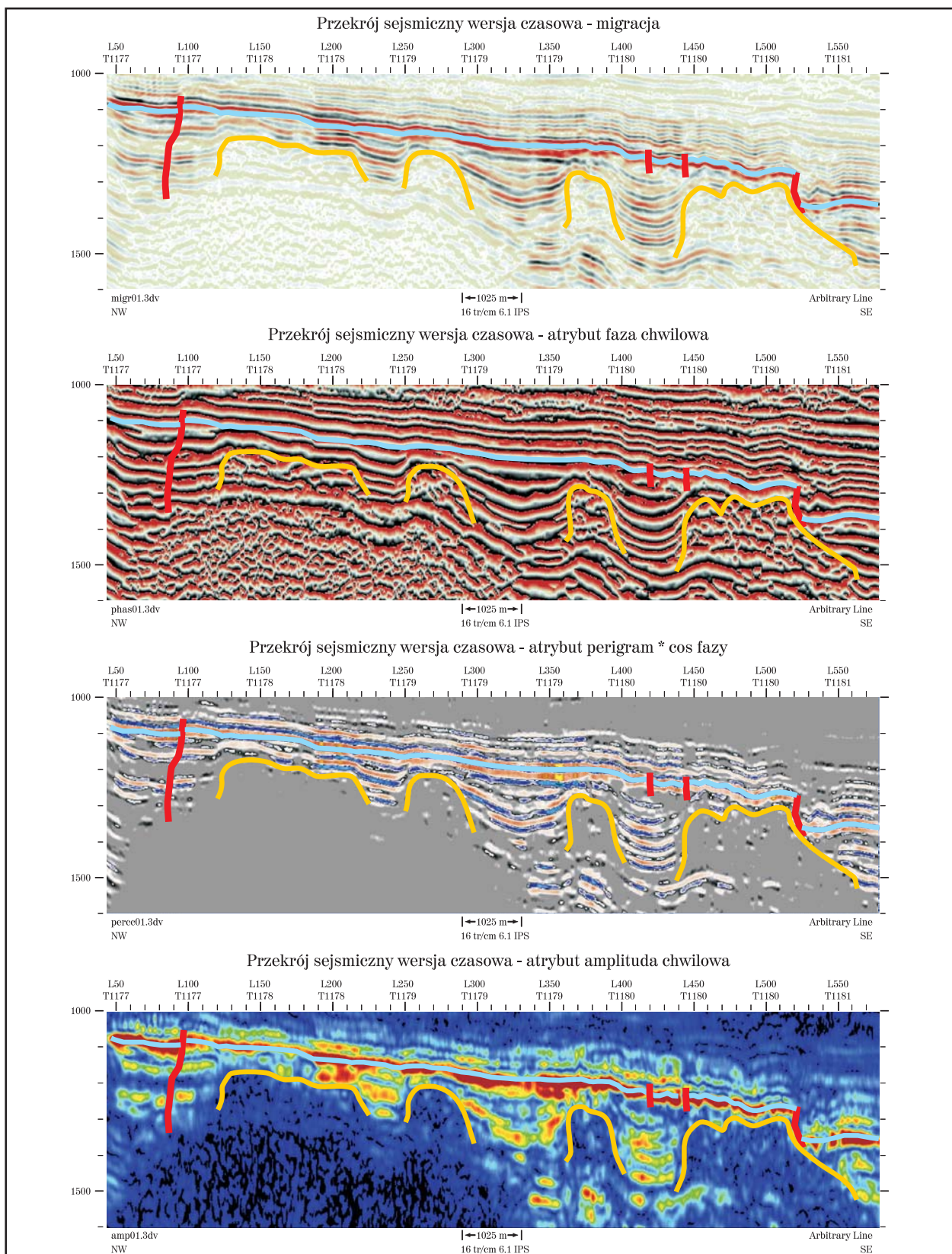
Fig. 3. Sekwencja biohermowa w zapisie sejsmicznym (objaśnienia jak na fig. 2).
